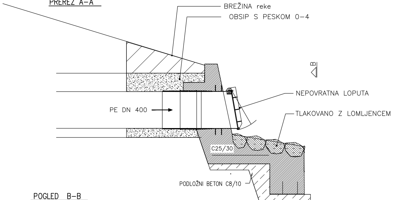
PREREZ A-A
