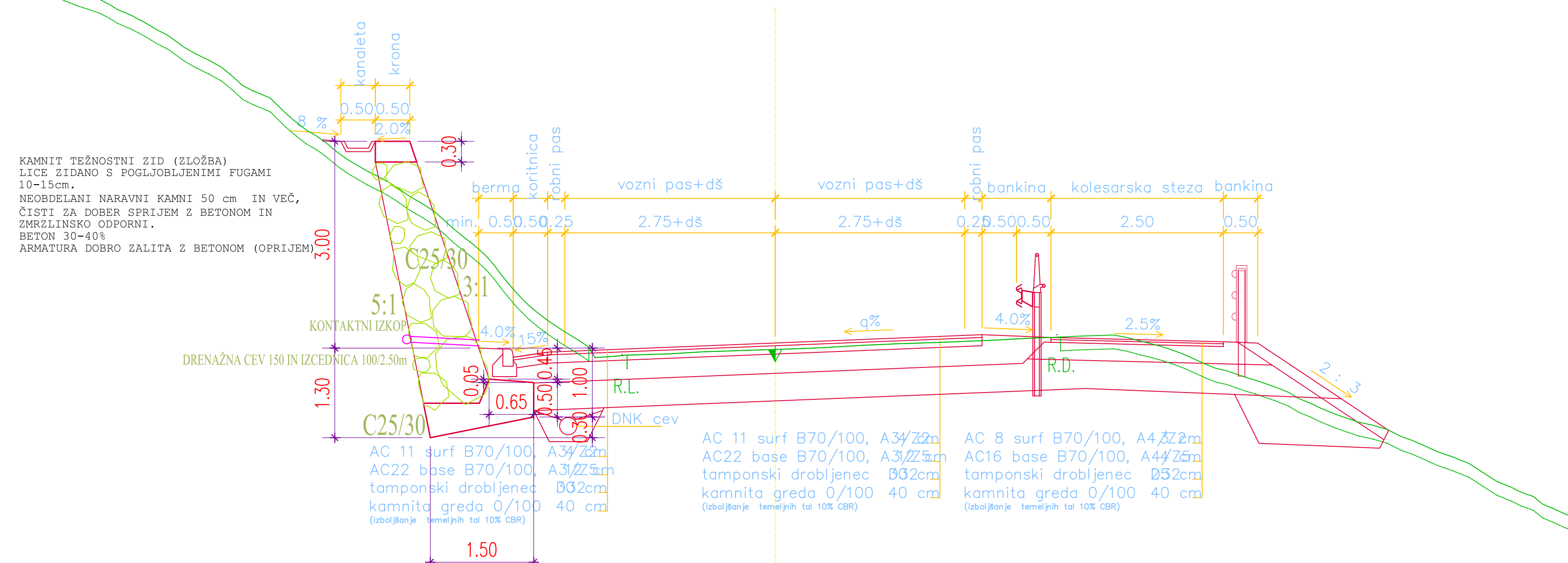
KARAKTERISTIČNI PREREZ odsek od km 3,297 do km 3,397
