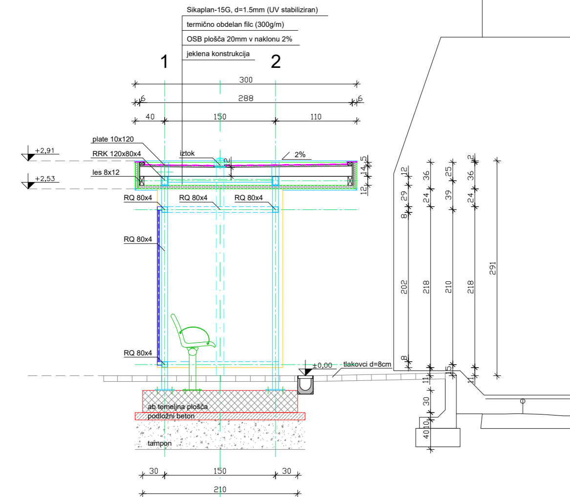
PREČNI PREREZ A - A
