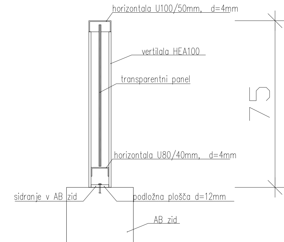
PREČNI PREREZ M 1:10
